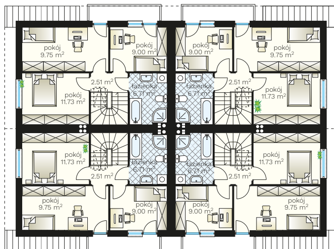
piętro > 39,70 m 2
