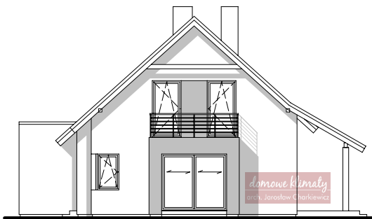
ELEWACJA PRAWA
