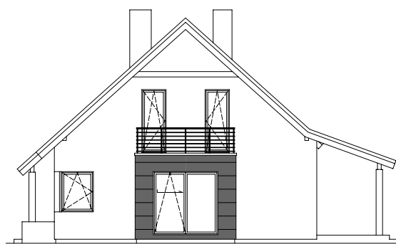
ELEWACJA PRAWA
