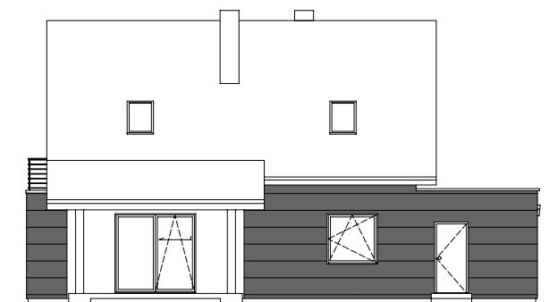
ELEWACJA OGRODOWA
