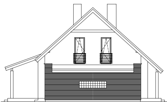
ELEWACJA LEWA
