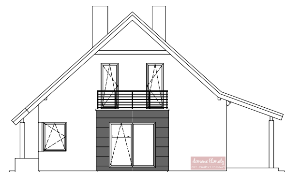
ELEWACJA PRAWA
