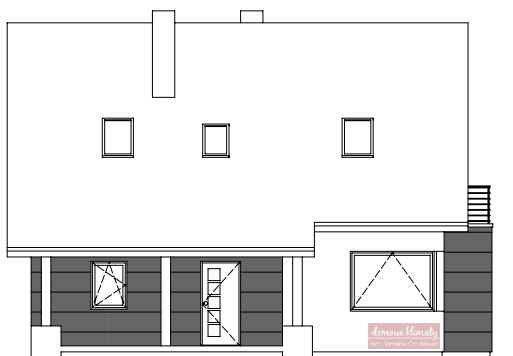
ELEWACJA FRONTOWA
