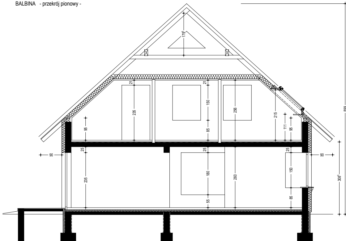
BALBINA - przekrój pionowy -
