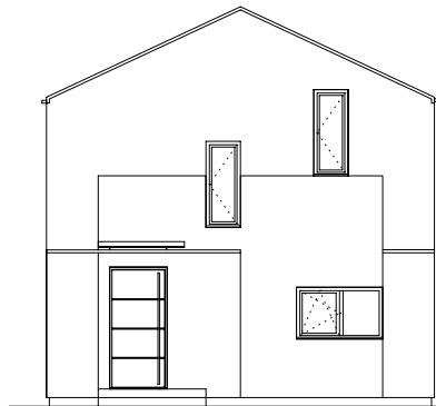
ELEWACJA FRONTOWA
