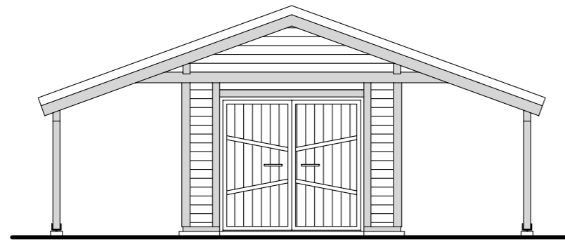
ELEWACJA FRONTOWA
