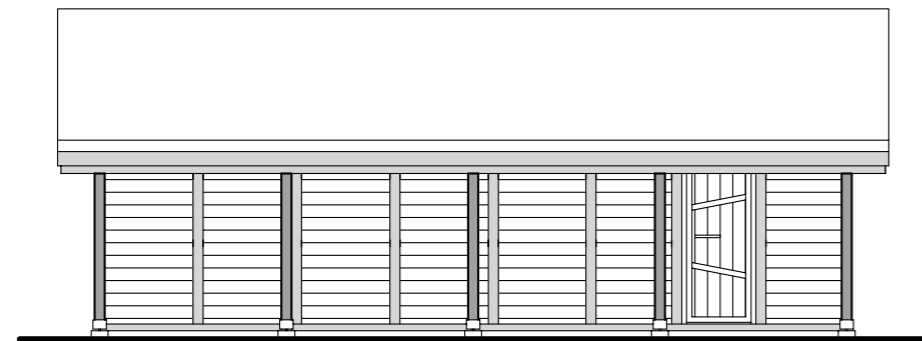
ELEWACJA PRAWA
