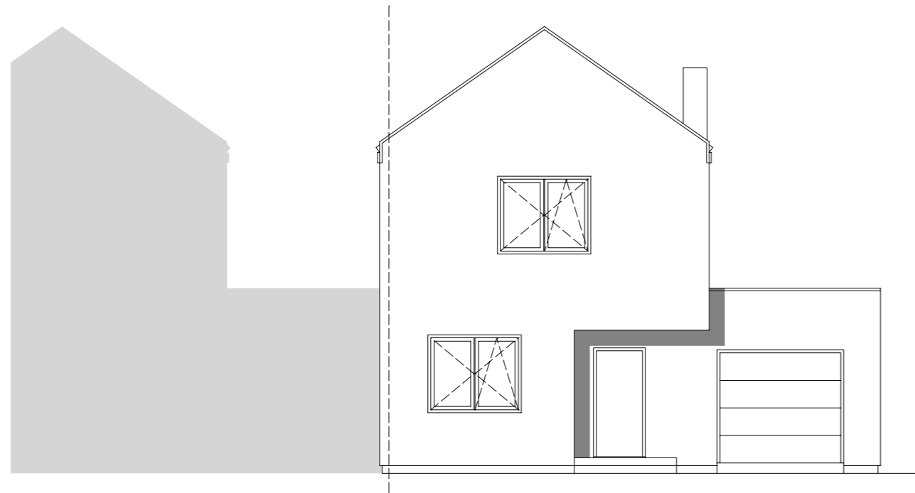
ELEWACJA FRONTOWA
