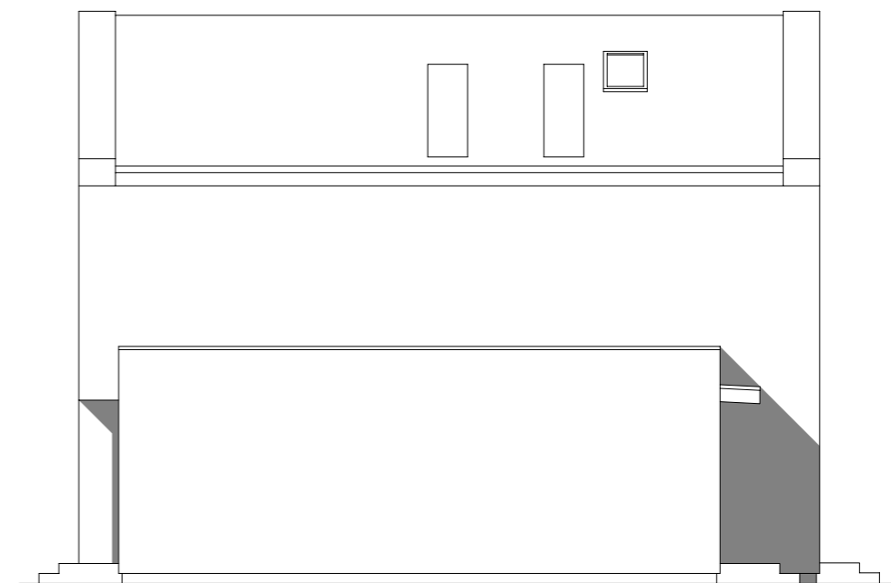
ELEWACJA LEWA
