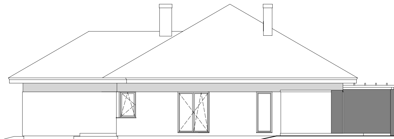
ELEWACJA PRAWA
