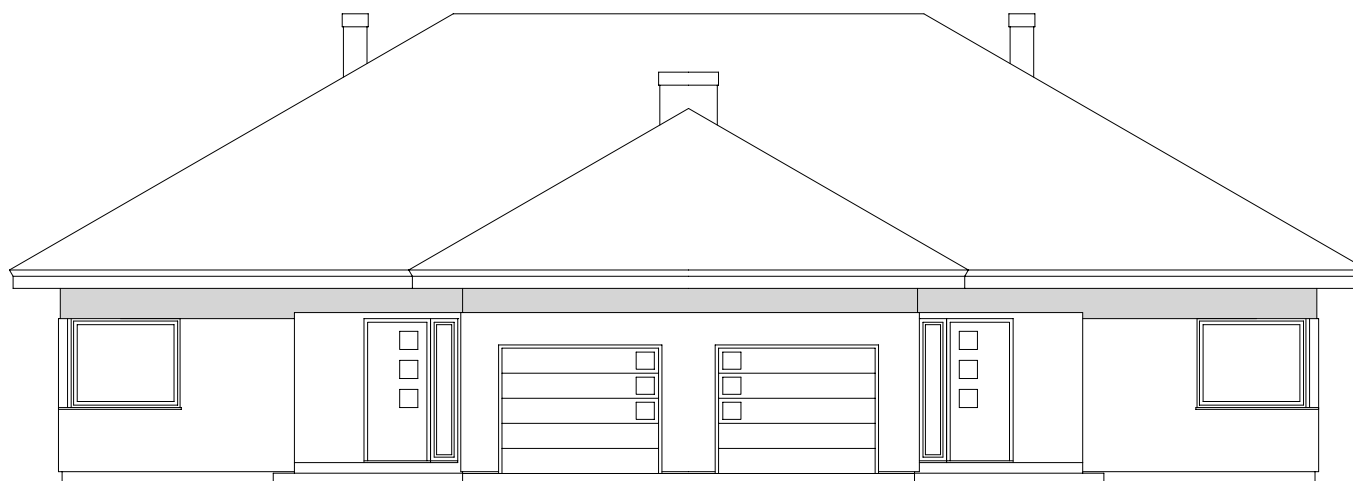
ELEWACJA FRONTOWA
