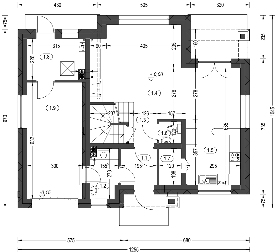
Zestawienie powierzchni parteru
