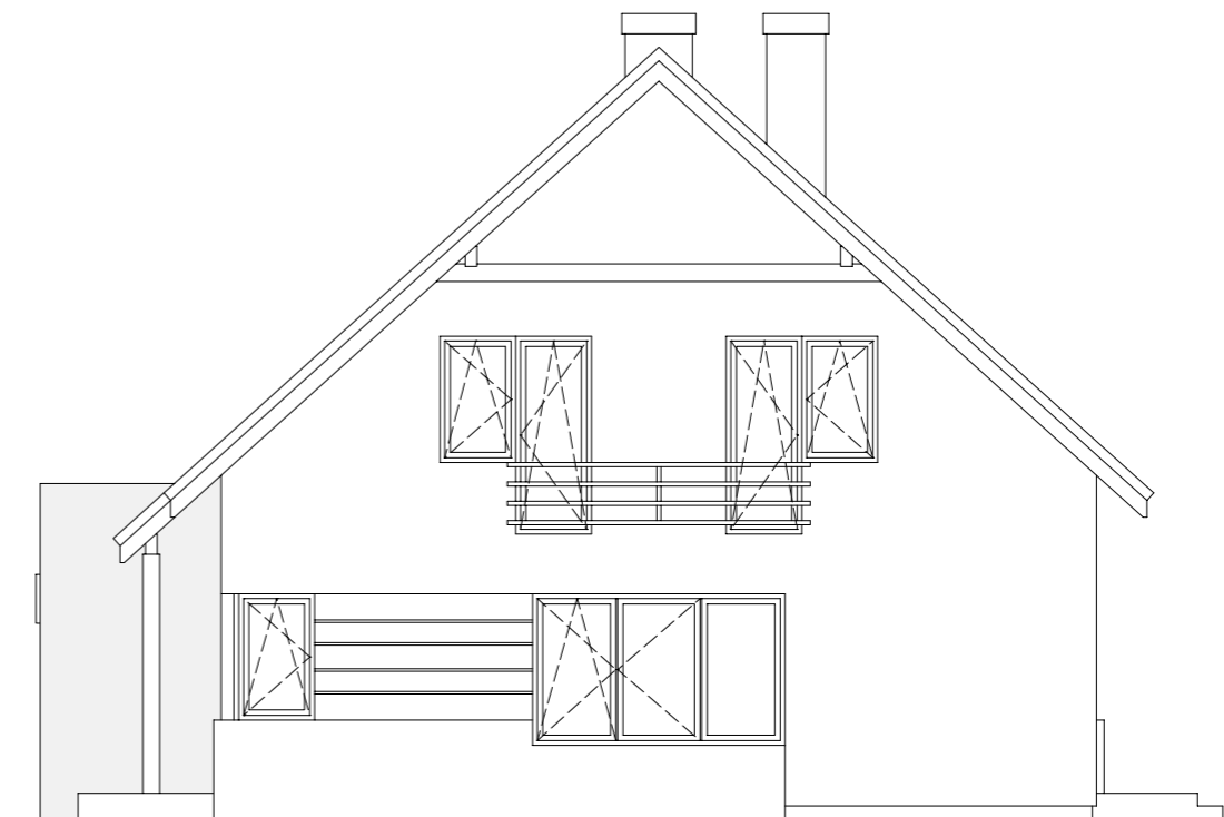
ELEWACJA PRAWA
