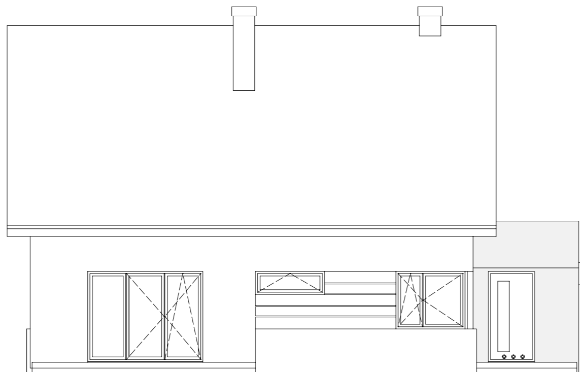
ELEWACJA OGRODOWA
