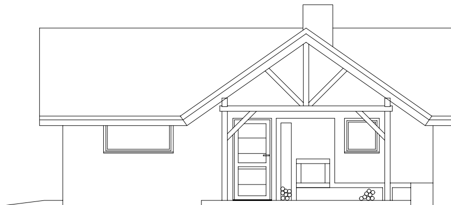
elewacja boczna
