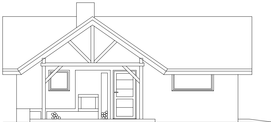
elewacja boczna
