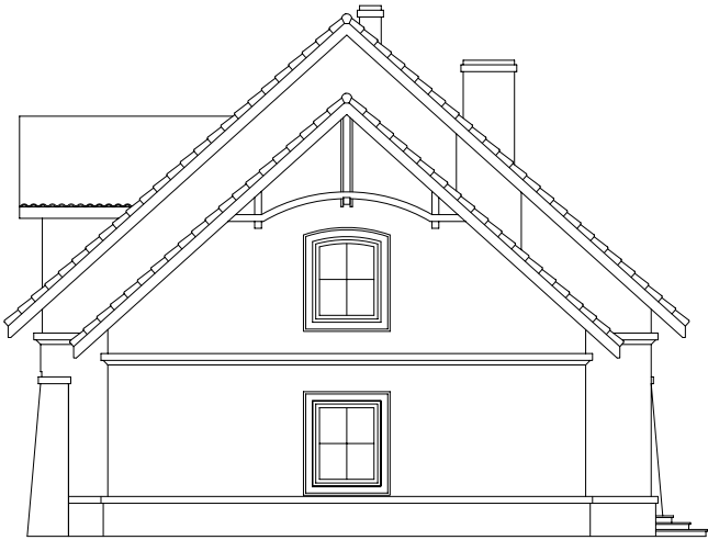
ELEWACJA PRAWA
