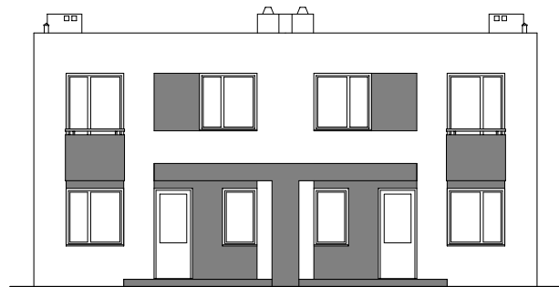
ELEWACJA FRONTOWA
