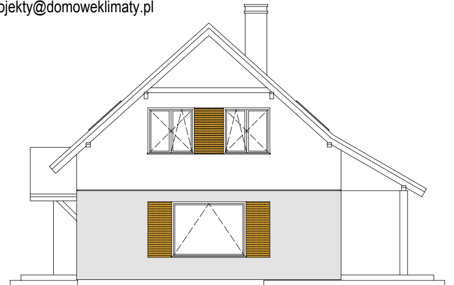
ELEWACJA BOCZNA PRAWA
